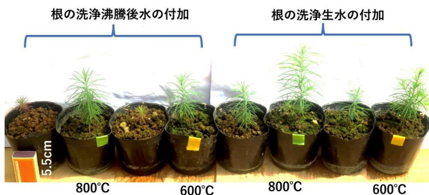
図-6. カラマツ芽生えの成長に及ぼす骨炭と根洗浄水の影響（約 135 日目） 800℃：生成時温度 800℃の牛骨炭；600℃：生成時温度 800℃の鶏骨炭。 左のマッチ箱の高さ：5.5cm
