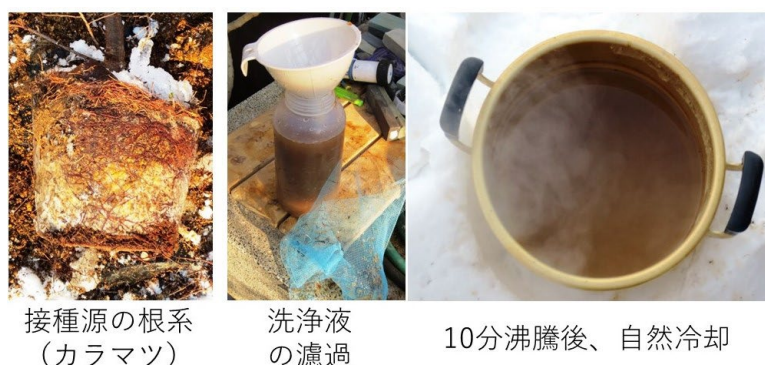
図-5. カラマツ根圏の洗浄液（接種源）
